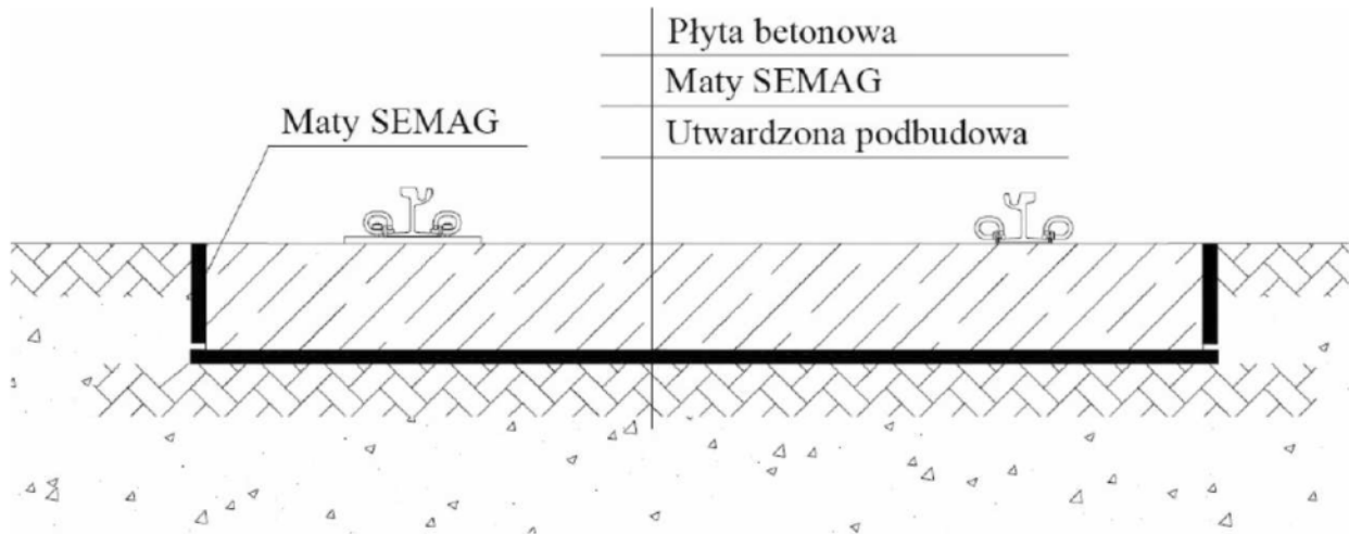
Rysunek Z-2 - Przekrój poprzeczny stosowania maty WM SEMAG w torowiskach o konstrukcji bezpodsypkowej
